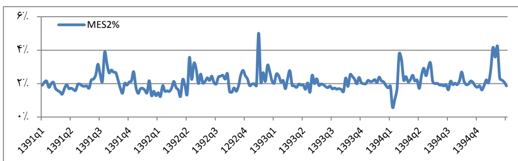
نمودار ۳. متوسط MES_{\%} در طول دوره نمونه
