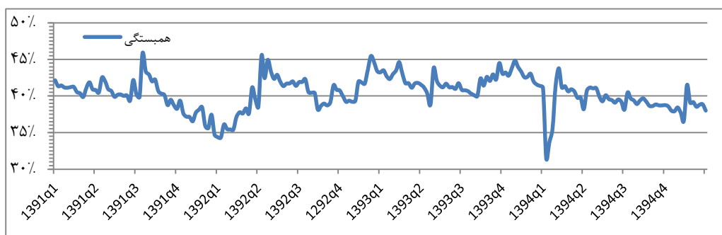
نمودار ۲. متوسط همبستگی‌ها در طول دوره نمونه
